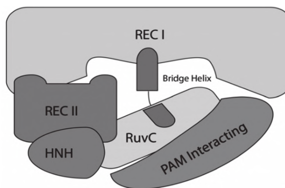
Рис. 1. Схема будови білка Cas9 у S. pyogenes [11,12].
