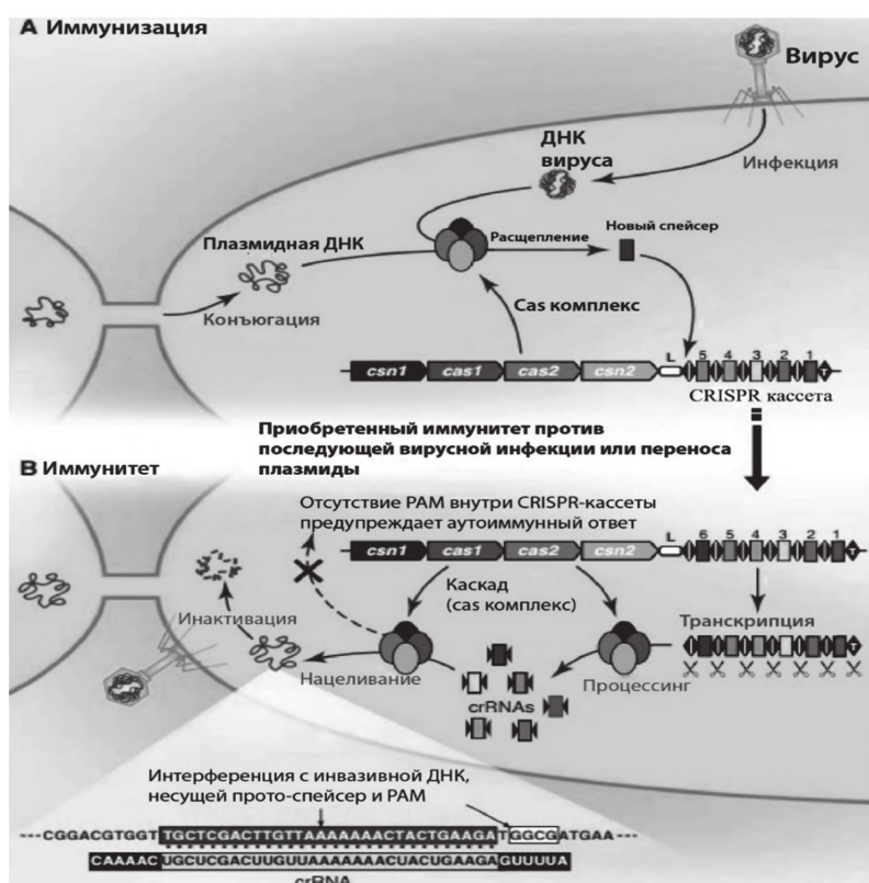
Рис. 3. Схема формирования иммунитета за допомогою системи CRISPR у Streptococcus thermophilus при інвазії плазмідної або вірусної ДНК [16,17].
